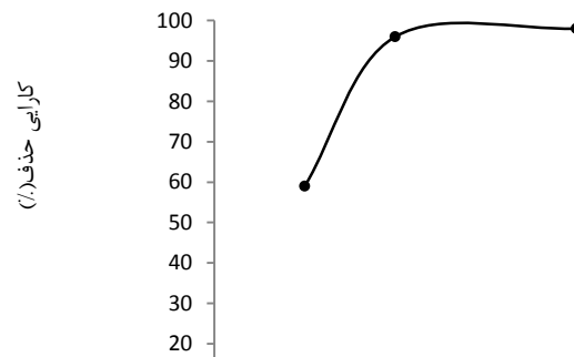
نمودار شماره ۳: تاثیر دوز جاذب بر کارایی حذف ۴و۲ دی نیترو فنل توسط CMK-3 (غلظت ۴و۲ دی نیترو فنل ۱۰۰ میلی گرم، زمان تماس ۱۰۰ دقیقه، pH=۵)
