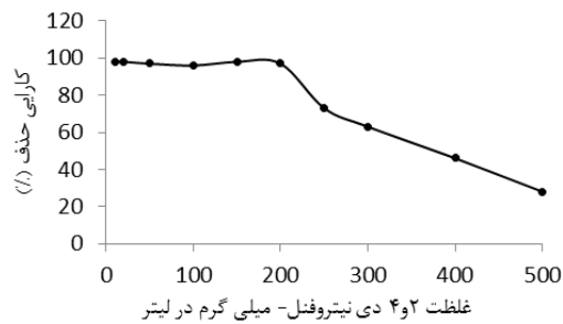
نمودار شماره ۴: تاثیر غلظت اولیه ۴و۲ دی نیترو فنل بر فرآیند جذب (pH 5، دوز جاذب ۰/۴ گرم در لیتر و زمان تماس ۱۰۰ دقیقه)
